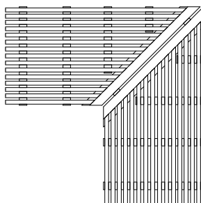
Gehrungsecke Art. Nr.: R51100 Parallelrost 250 mm breit
