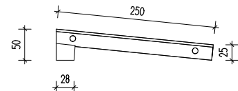
Art. Nr.: R30100 Schräger Querrost 250 mm breit
