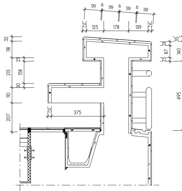
Schnitt/Coupe/Section/Sezione
