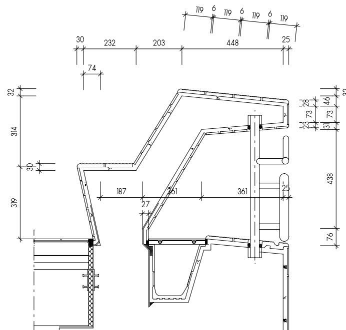
Schnitt/Coupe/Section/Sezione
